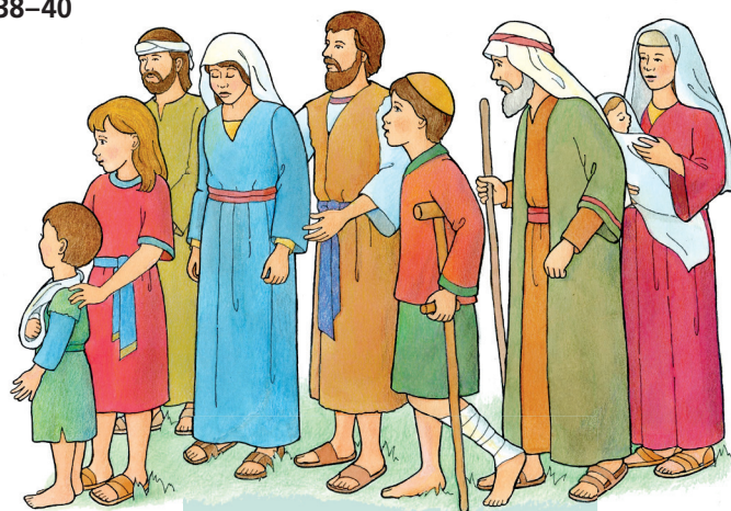
množica
